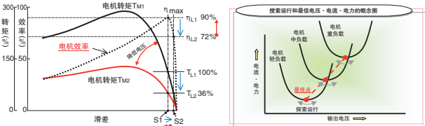
电机的滑差-转矩·效率特性 通用电机: 380V 7.5kW 4P
