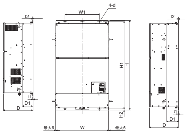
外形图 4
