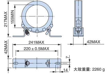
型号 F200160PB
