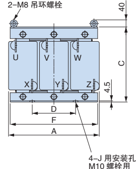
外形图 3
