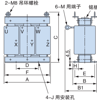
外形图 2
