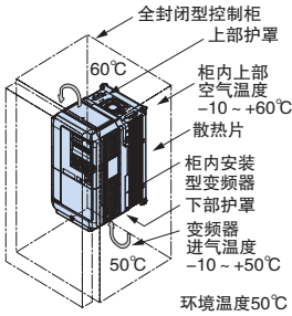
· 全封闭型控制柜内的安装图
