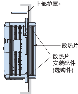
· 散热片外置安装图
