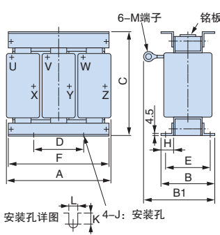
外形图 1
