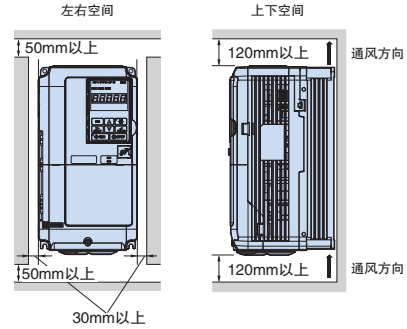
· 确保变频器的安装空间
