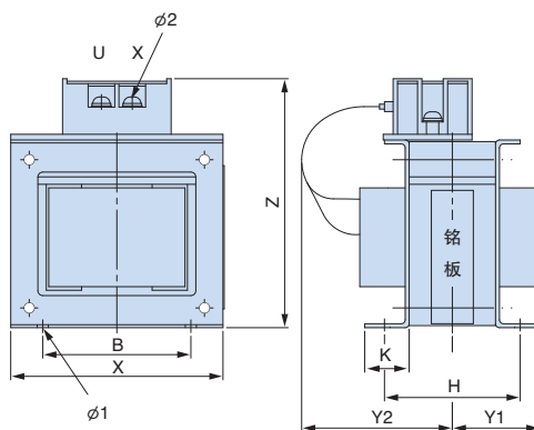
外形图 2
