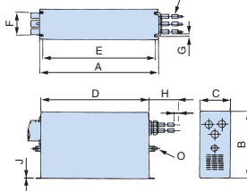
外形图3
