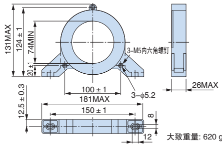
型号 F11080GB
