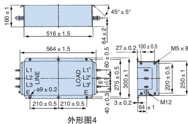
外形图4
