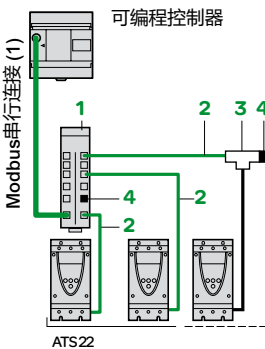
通过分接盒、RJ45连接器连接的Modbus串行连接实例
